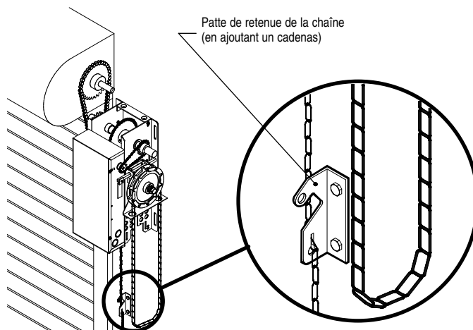
Verrouillage électrique avec palan du modèle MH
